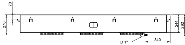
lado posterior
